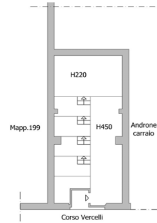
PIANTA SOPPALCO
